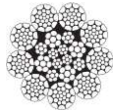
9-SR - за количките на кранове POTAIN
