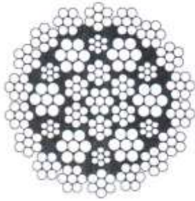
37x7 HERCULES
