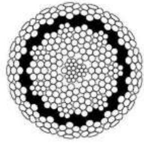
Hoist-C PYTHON с компактизирани телчета+екструдирана пластмаса
