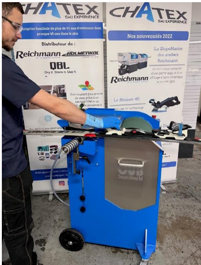
Заточване на страничен ъгъл на канта
