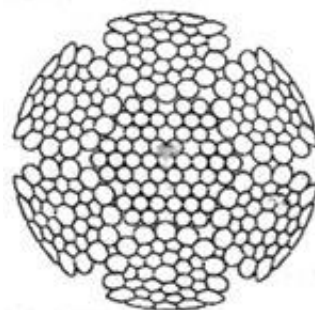
Същото въже след специална обработка по профилиране на външните телове - конструкция тип Python
