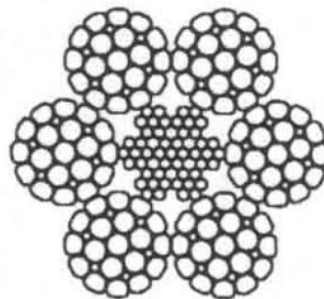
Стандартно въже с конструкция 6x25+стоманена сърцевина
