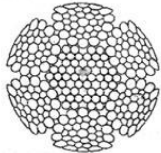
Същото въже след специална обработка по профилиране на външните телове - конструкция тип Python
